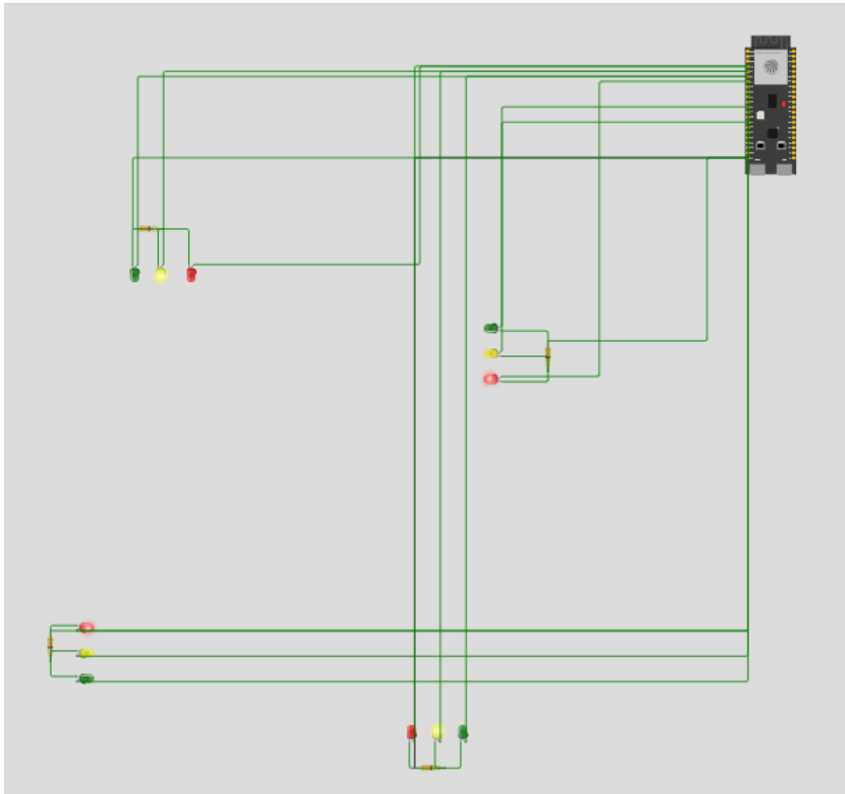
Hình 3. Sơ đồ mạch ESP32.
